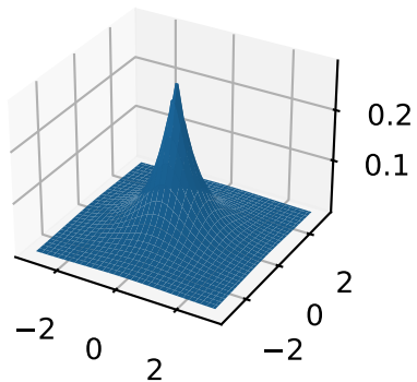
'exponential', 2-norm
