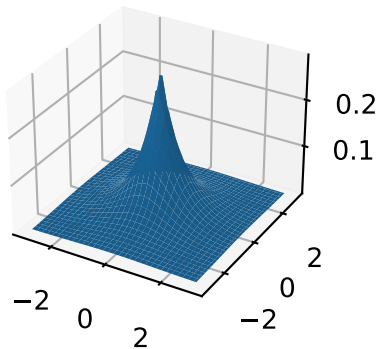
'exponential', 2-norm
